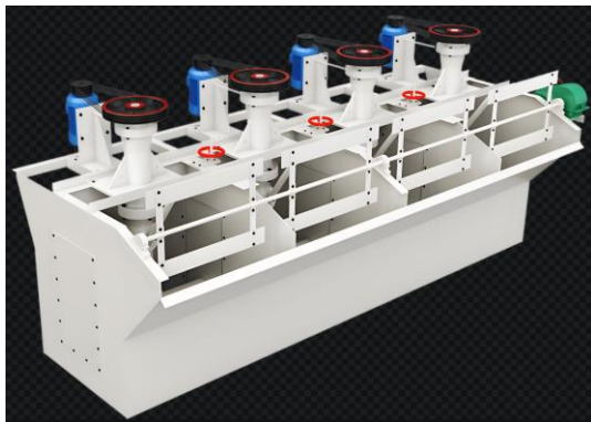
دستگاه فلو تاسیون
